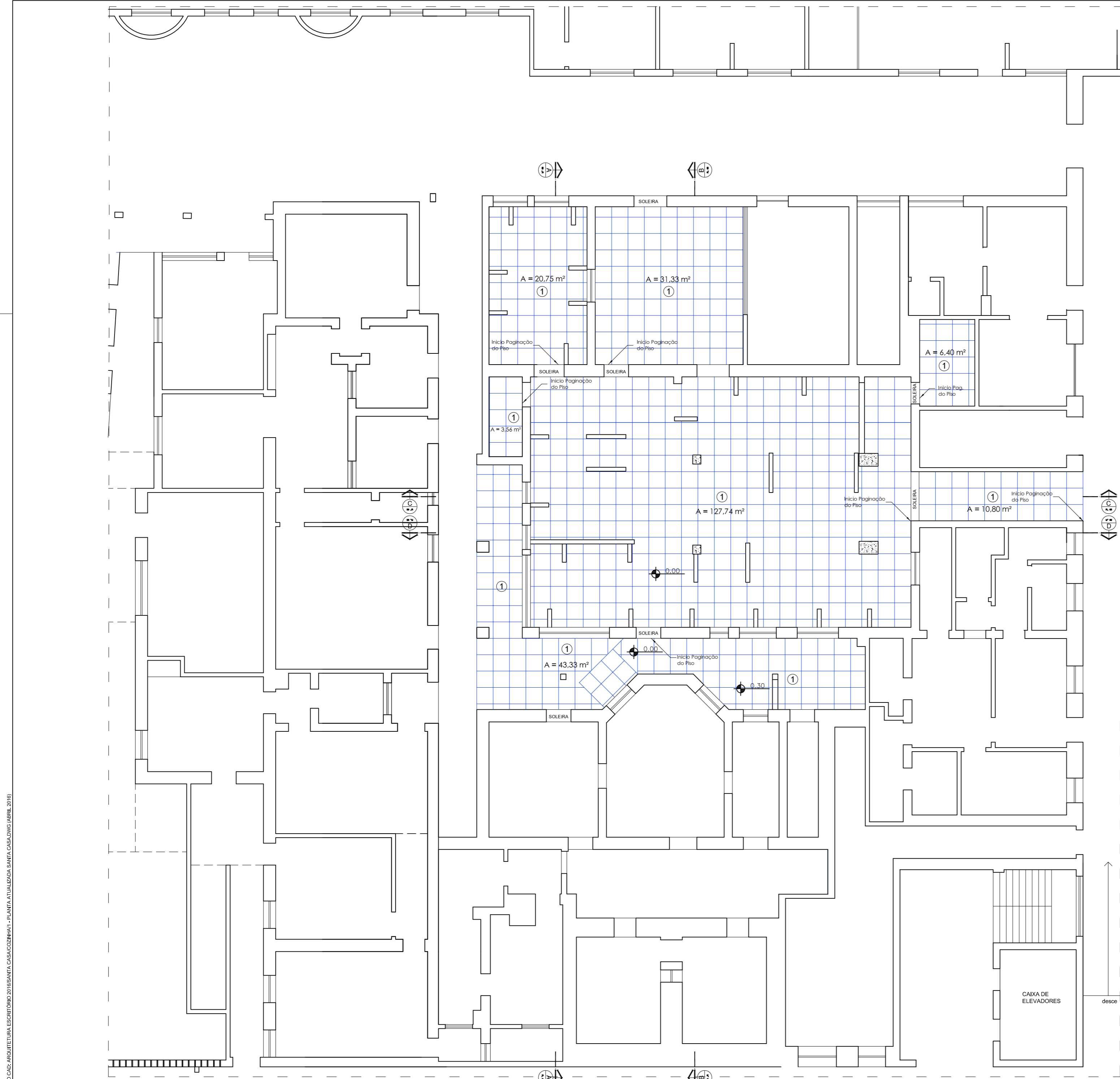
PLANTA BAIXA PAV. TÉRREO - (PISO A EXECUTAR) ÁREA TOTAL DE PISO 243,91 M² escala 1:100
