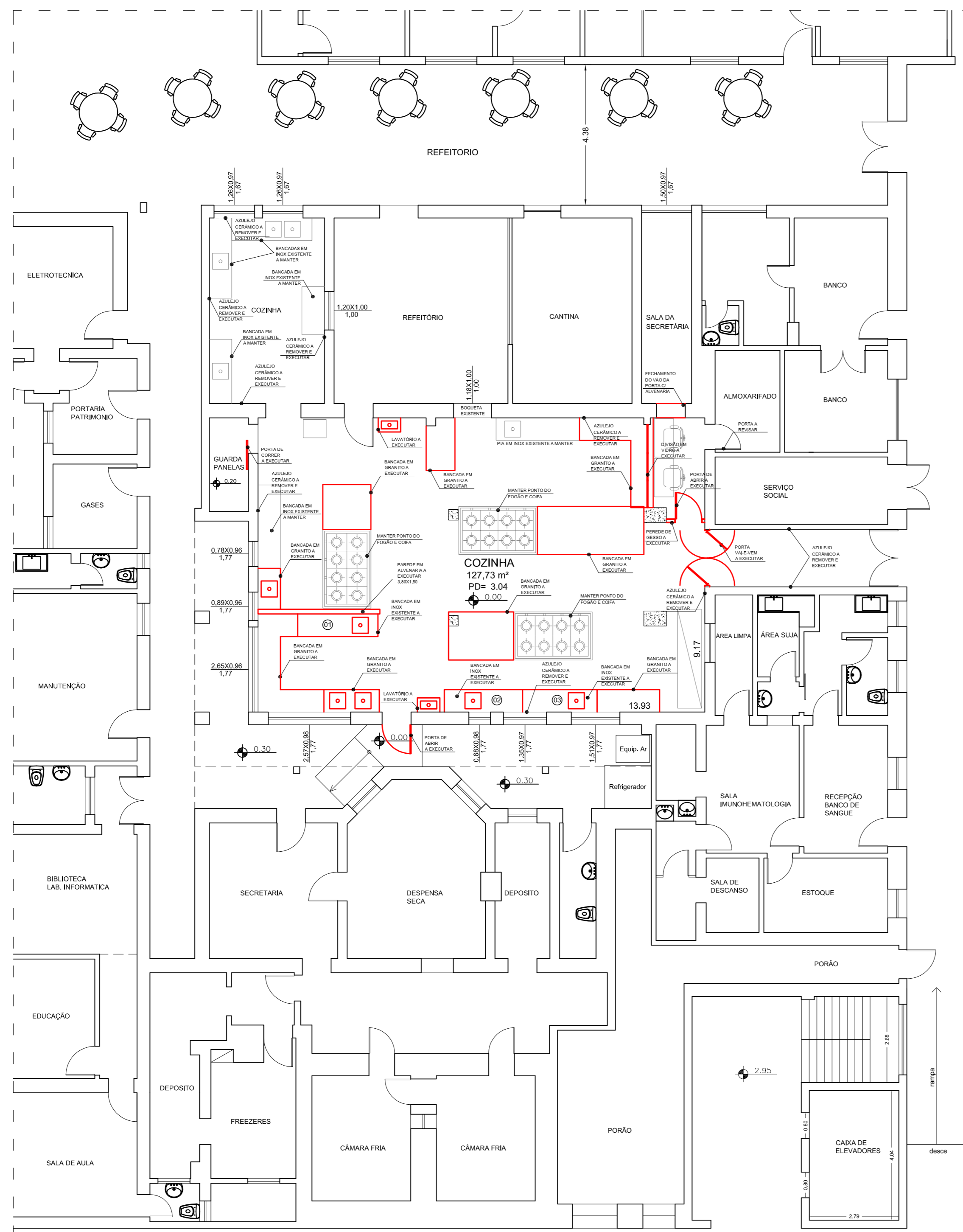
PLANTA BAIXA PAV. TÉRREO- (A CONSTRUIR) (PROPOSTA 02) escala 1:100
