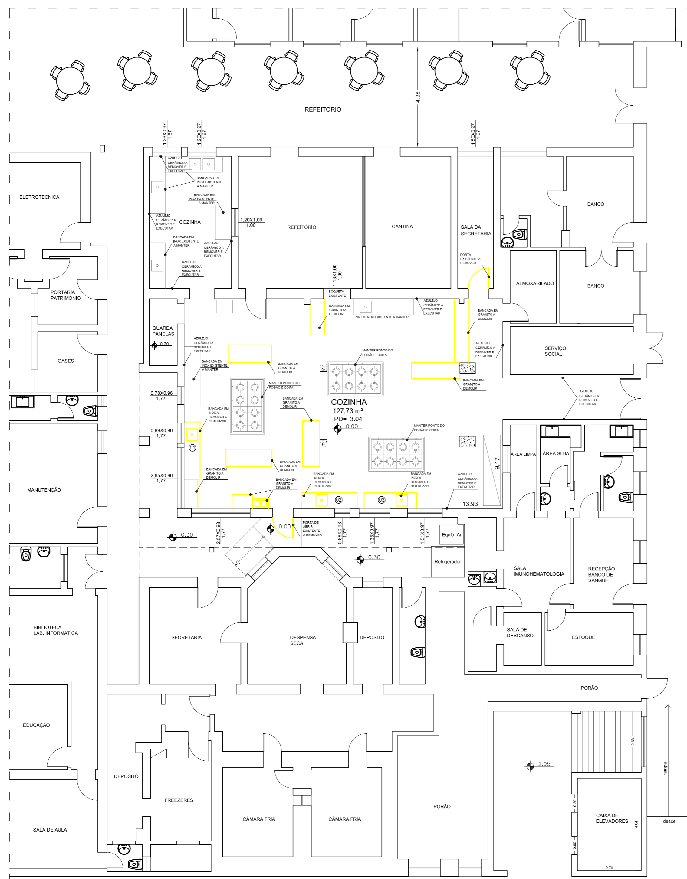
PLANTA BAIXA PAV. TÉRREO- (A DEMOLIR) (PROPOSTA 02) escala 1:100
